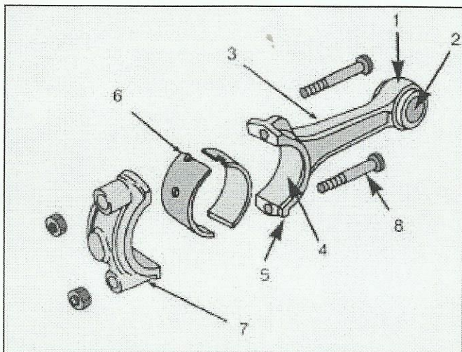
Σχήμα 3.2.3 Μέρη διωστήρα (μπιέλα)
