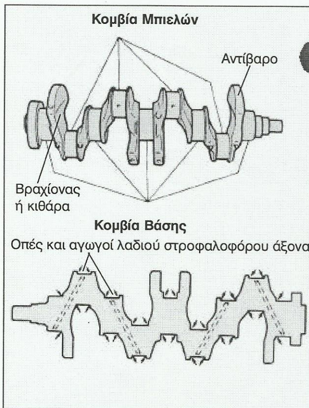
Σχήμα 3.2.4 Μέρη ενός στροφαλοφόρου άξονα
