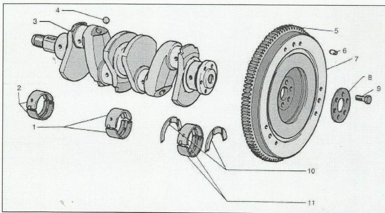
Σχήμα 3.2.5 Στροφαλοφόρος άξονας και σφόνδυλος (βολάν)
