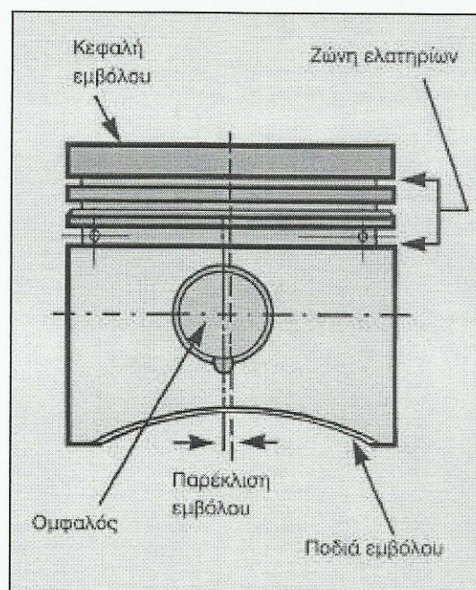
Σχήμα 2.2.2 Τα τμήματα του εμβόλου
